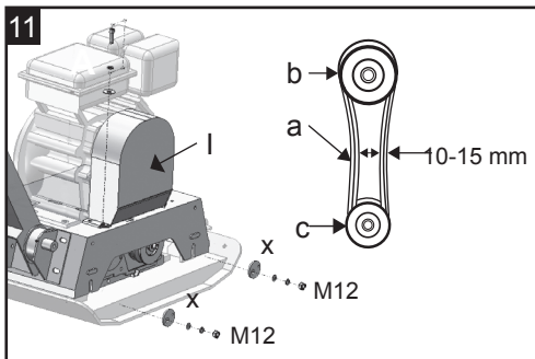
Antriebsriemen
