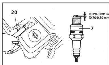
Zündkerze
