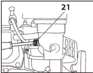
Drosselanschlagschraube
