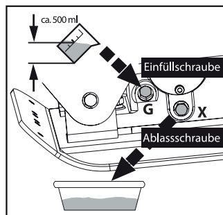
Erregeröl wechseln
