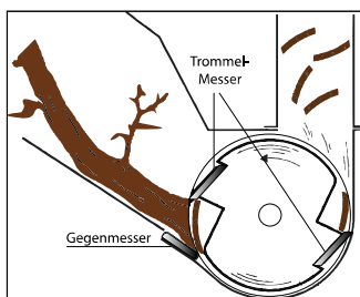
Duplex-Messertrommel
