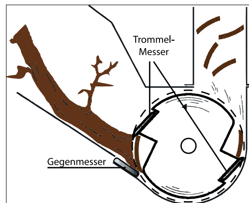
Trommelhackwerk
