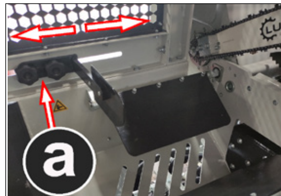
(a) Verstellbarer Anschlag mittels Sterngriffschrauben
